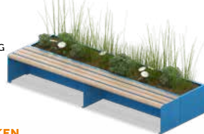
CC BANK LANG MIT BEET CC BENCH WITH PLANT BED LONG 14.02.897 ⊕ 3,00x 0,60 x 0,45 m
