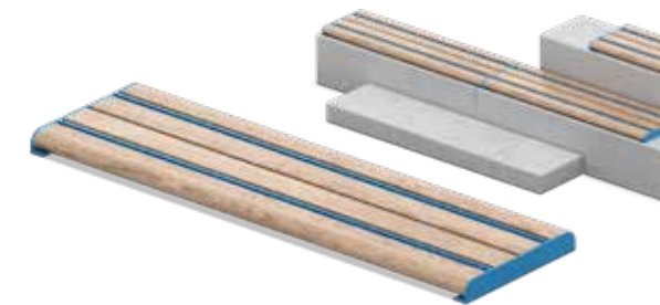
CC SITZAUFLAGE CC SEAT COVER 14.02.524 ⊕ 1,50 x 0,45 x 0,06 m
