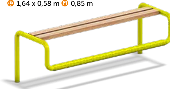
JUGENDBANK PULVERBESCHICHTET TEEN BENCH POWDERCOATED 14.01.010.004 ⊕ 1,64 x 0,58 m ⊕ 0,85 m
